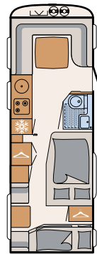
650 RFK 7 slaappleaatsen
