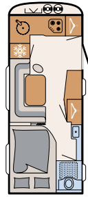
490 BLF 3 slaappleaatsen
